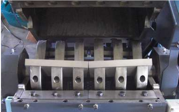
粉碎室内部
